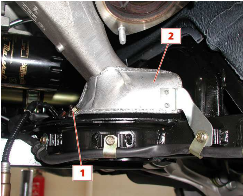
15. 安装发动机下端的防护装置。
